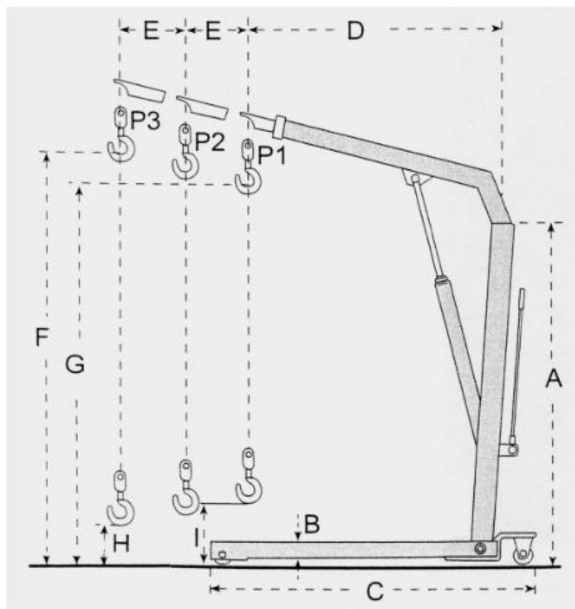
Abmessungen mm
